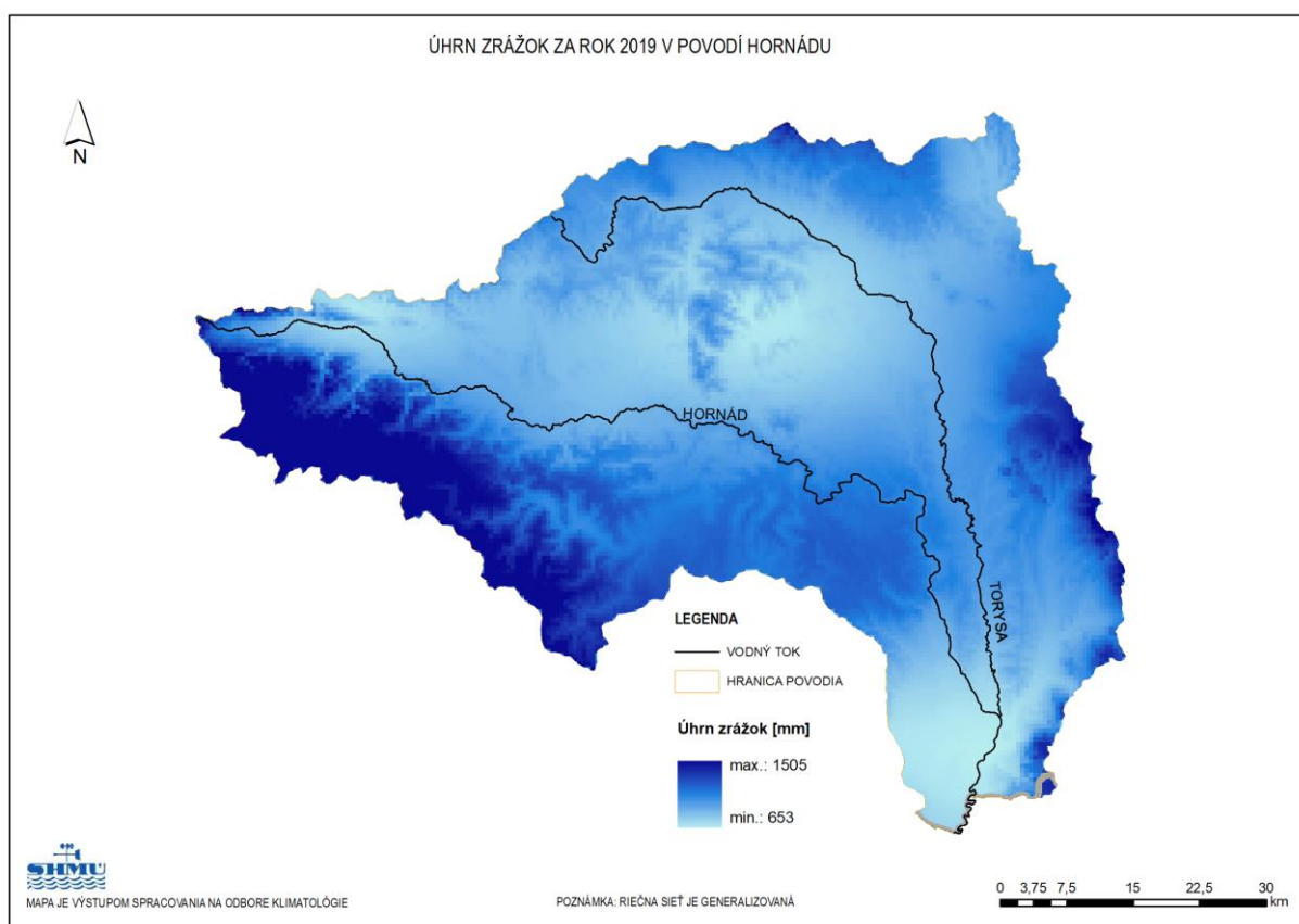
Obr. 4.2. Úhrn zrážok v povodí Hornádu v roku 2019
