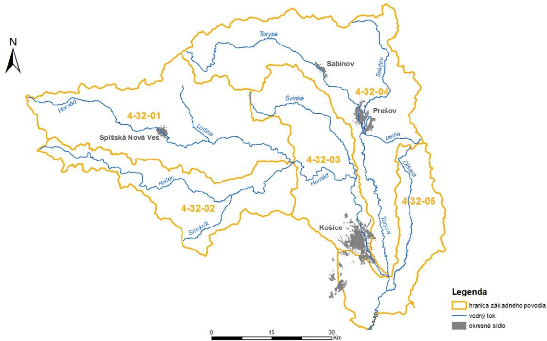
Obr. 2.2. Čiastkové povodie Hornádu
