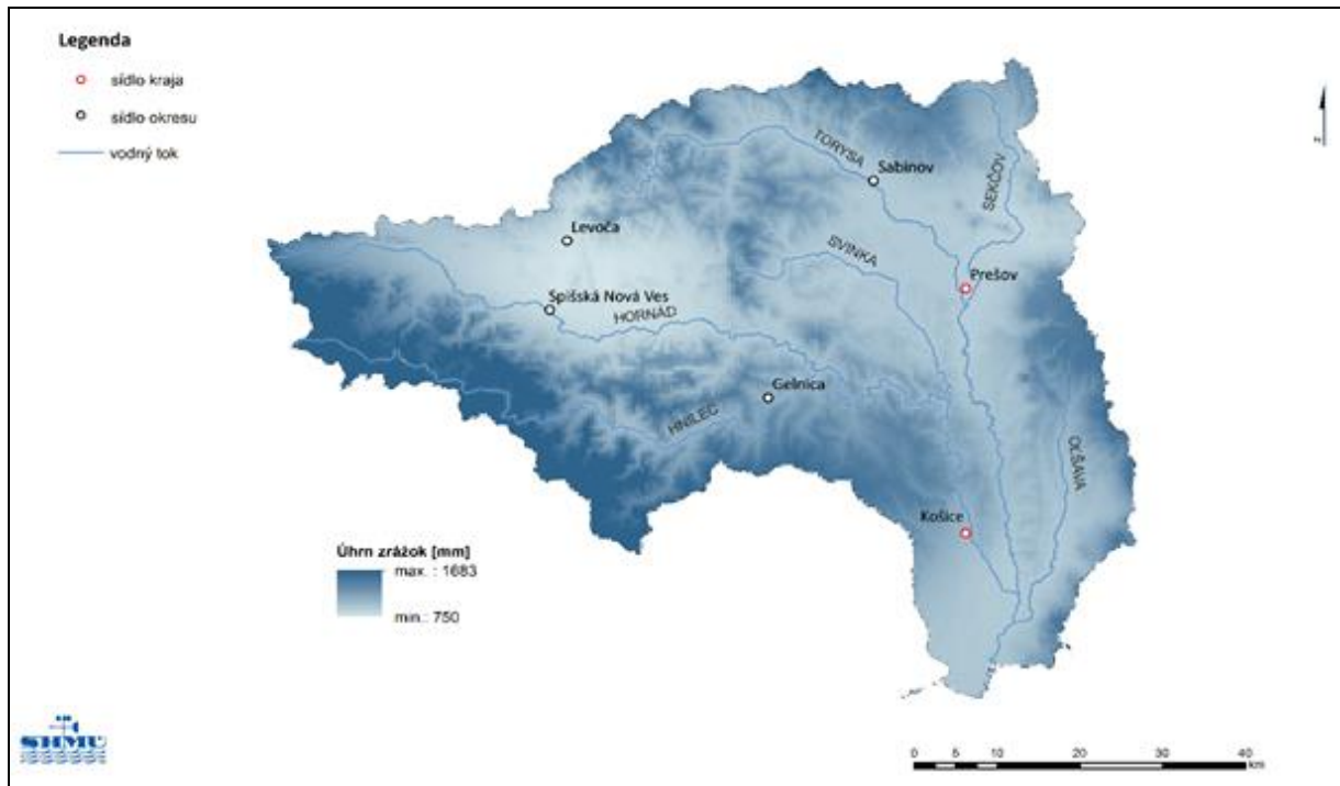
Obr. 4.6. Úhrn atmosférických zrážok v povodí Hornádu za rok 2023
