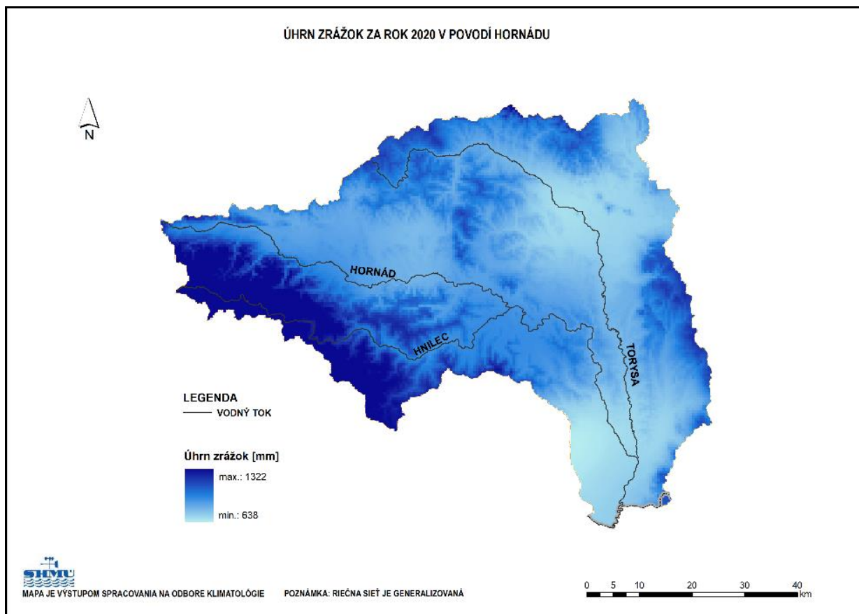
Obr. 4.3. Úhrn zrážok v povodí Hornádu za rok 2020
