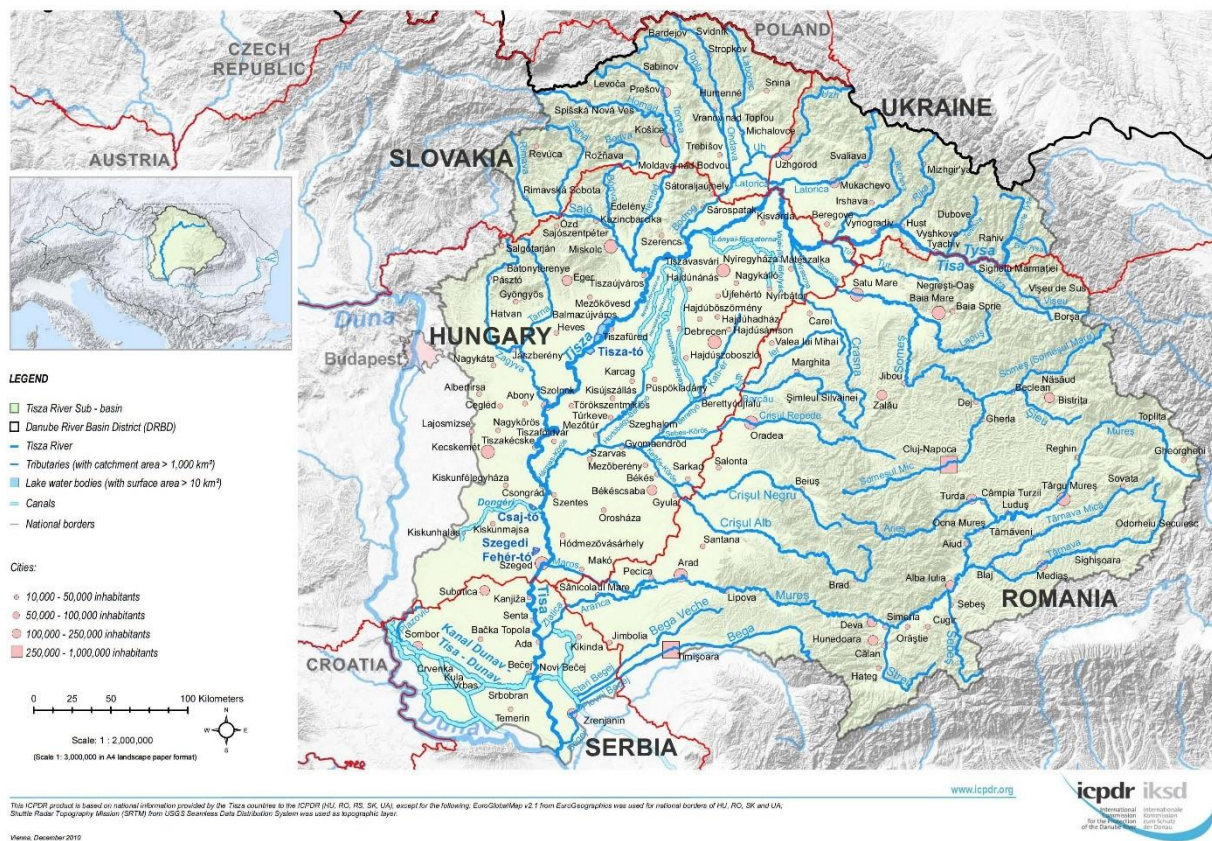
Obr. 3.2. Medzinárodné čiastkové povodie Tisy [237]
