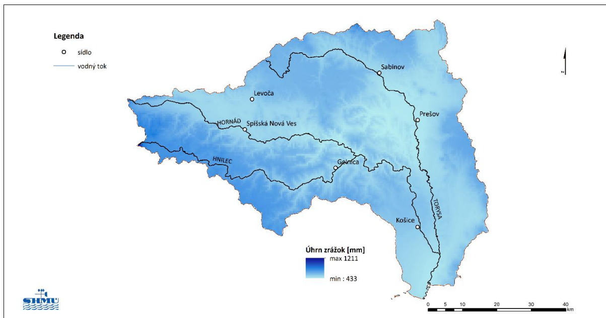
Obr. 4.5. Úhrn atmosférických zrážok v povodí Hornádu za rok 2022
