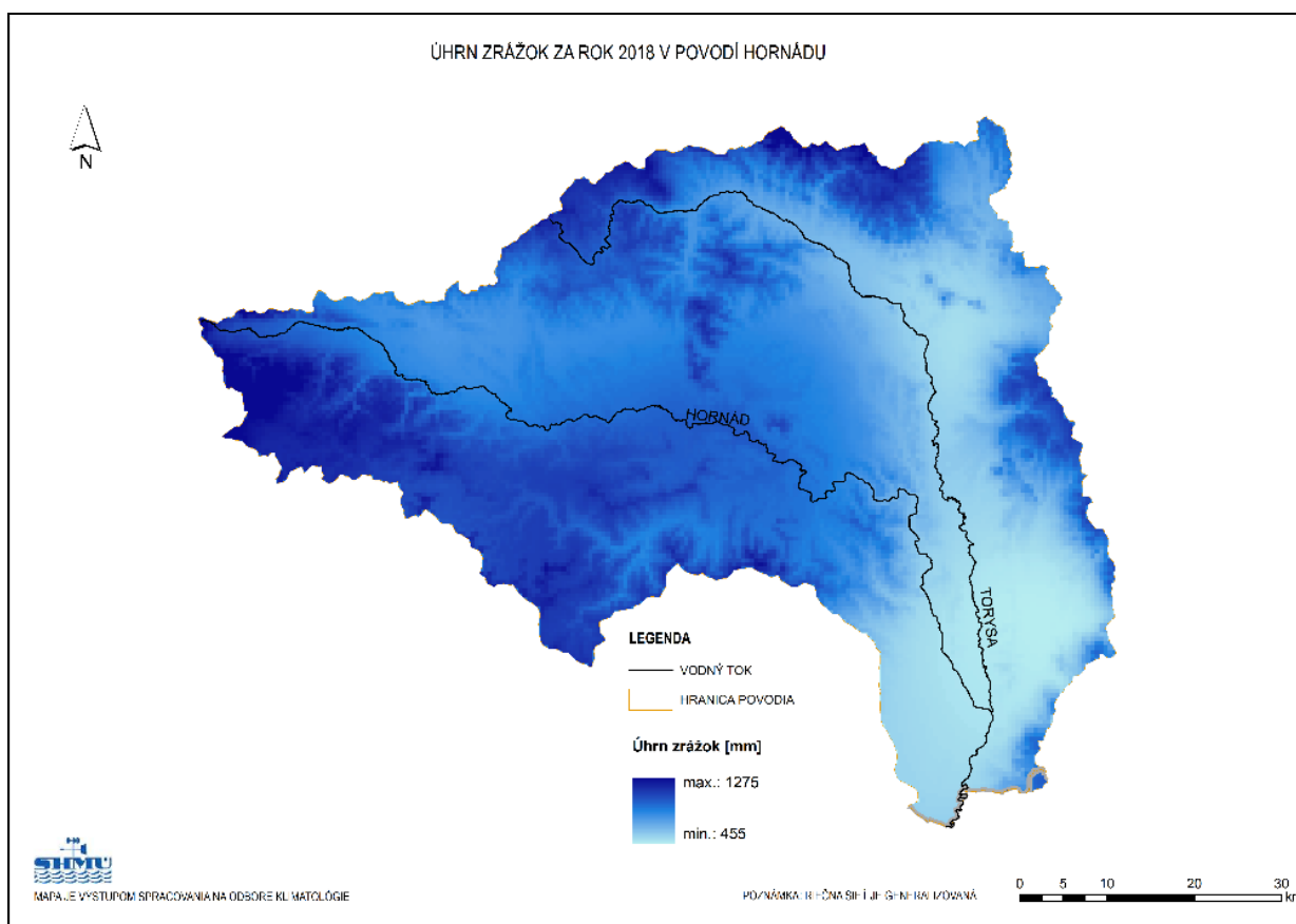
Obr. 4.1. Úhrn zrážok v povodí Hornádu v roku 2018
