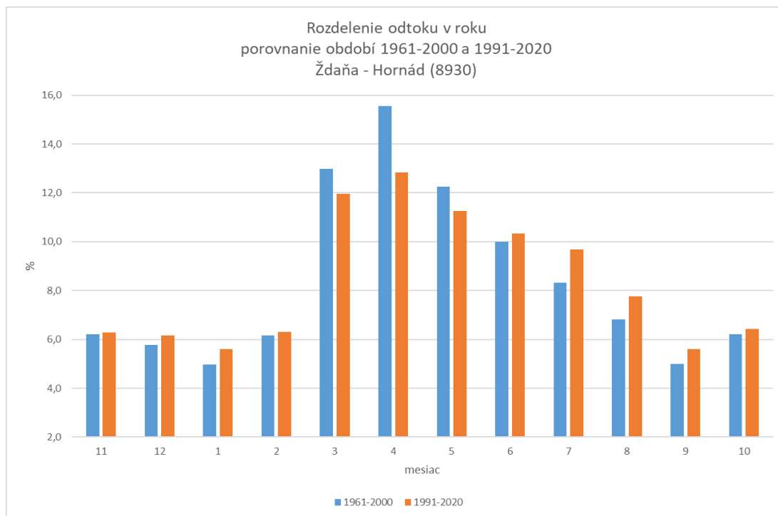
Obr. 3.3. Zmeny rozdelenia odtoku v roku obdobia 1991-2020 voči obdobiu 1961-2000, VS Ždaňa - Hornád
