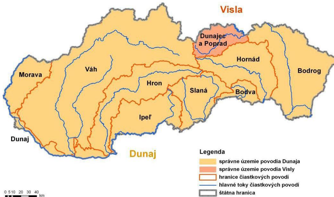
Obr. 1.1. Správne územia povodí na území Slovenskej republiky a ich čiastkové povodia
