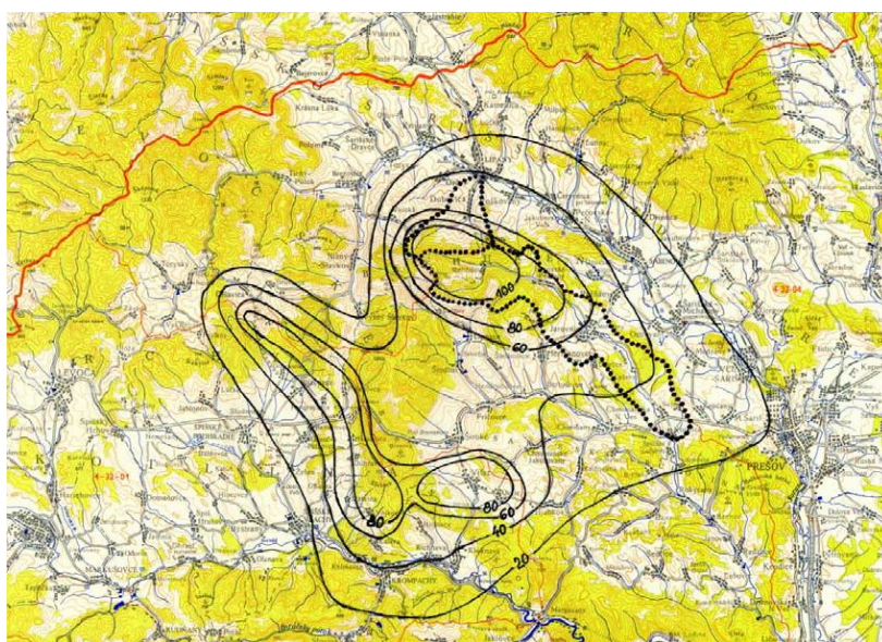
Obr. 4.9. Rekonštrukcia izohyet extrémneho dažďa, ktorý spôsobil 20. 7. 1998 prívalovú povodeň v Malej Svinke a Dubovickom potoku [235]
