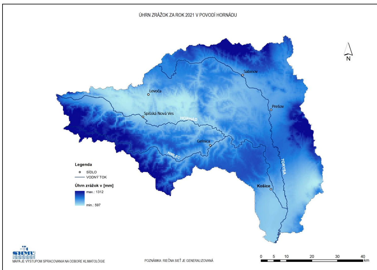
Obr. 4.4. Úhrn zrážok v povodí Hornádu za rok 2021
