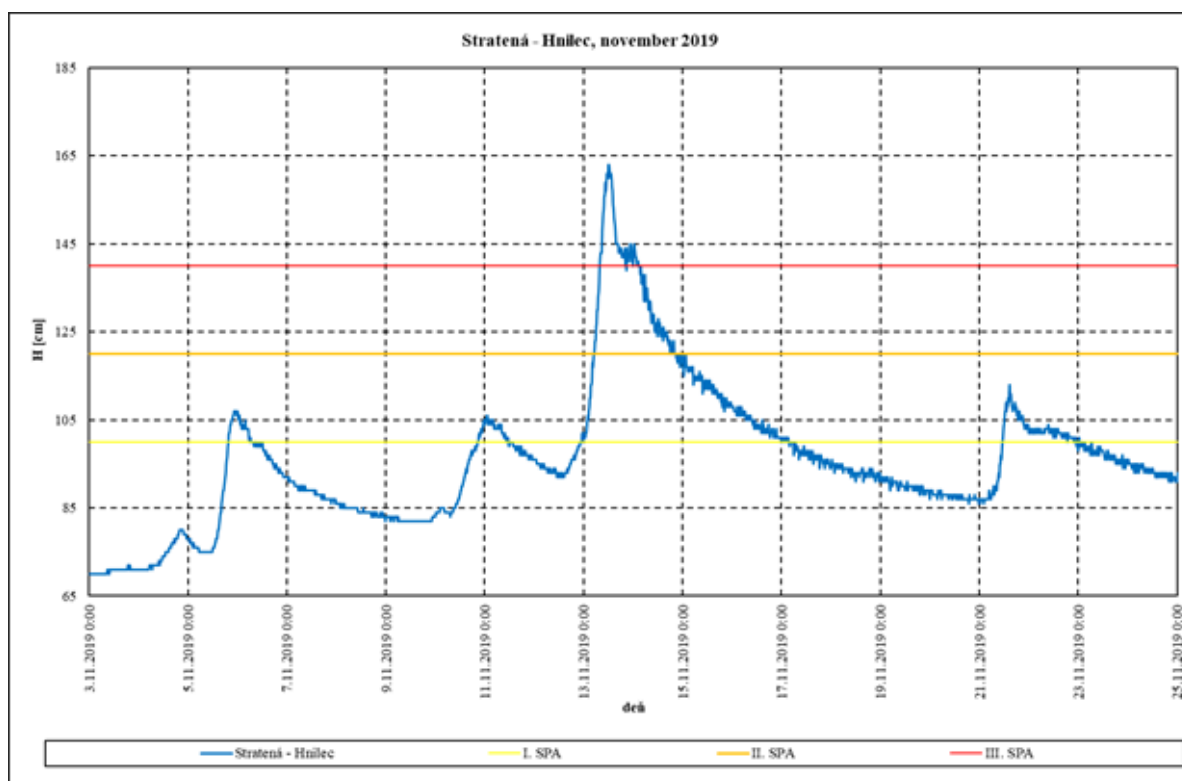
Obr. 4.10. Priebeh povodňovej situácie vo vodomernej stanici Stratená na Hnilci v novembri 2019
