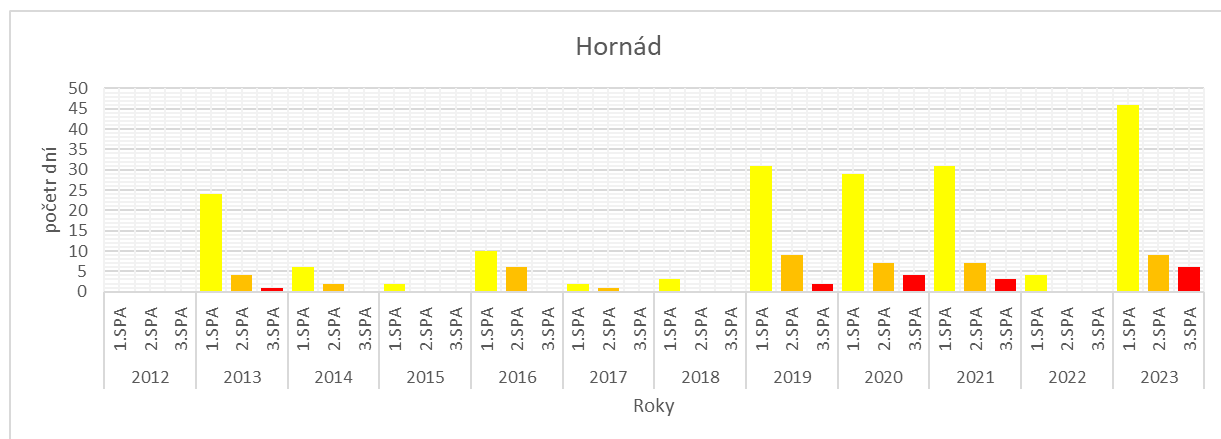
Obr. 4.11. Počet dní s výskytom 1.-3. SPA v povodí Hornádu
