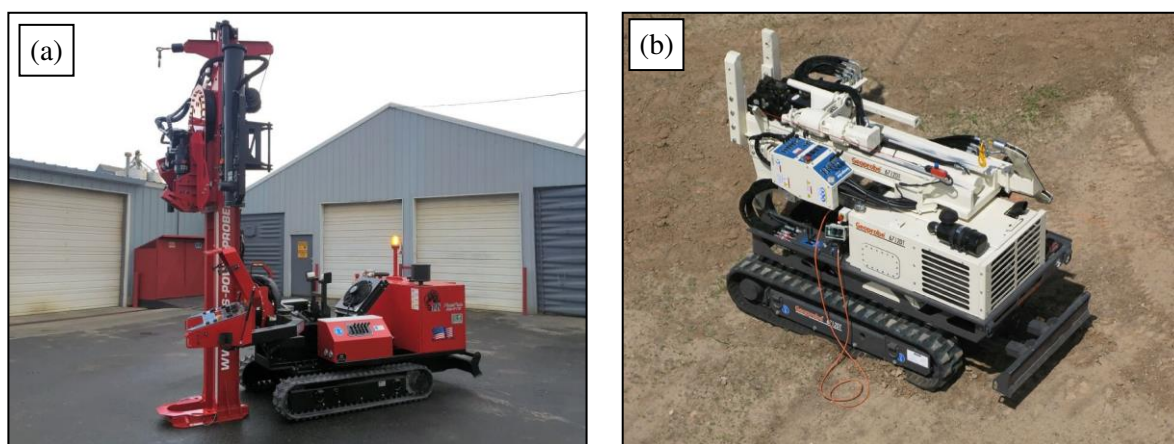
Obrázok 5. Vzorkovacie súpravy strednej triedy od sp. AMS (a) a Geoprobe® (b)
