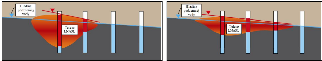
Obrázok P13_7. Vývoj tvaru kontaminačného mraku LNAPL vo vertikálnom reze a jeho prejavov vo forme voľnej fázy ropných látok na hladine podzemnej vody vo vrtoch v prevažne pórovom prostredí
