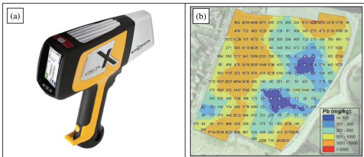
Obrázok 18. Ručný röntgenový analyzátor (XRF spektrometer DELTA) (a) a príklad jeho využitia na monoprvkovej mape Pb (krok merania 20 × 20m) (b)
