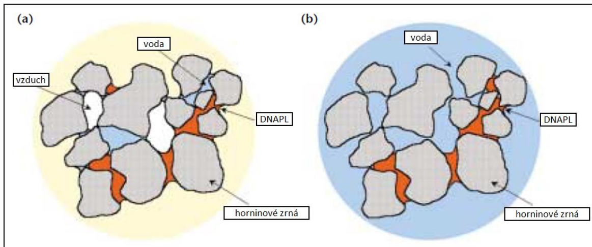
Obrázok P13_10. Reziiduálna voľná fáza látky ropného pôvodu ťažšej ako voda a jej správanie sa v pásme prevzdušnenia (a) a v pásme nasýtenia (b)
