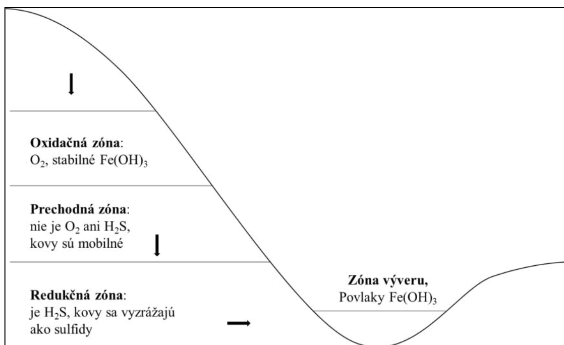
Obrázok P13_5. Koncepčný model transportu kovov
