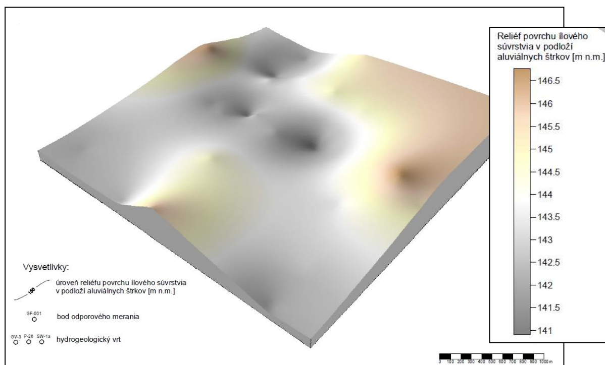
Obrázok 13. 3D vizualizácia reliéfu ílového podložja vytvorená na základe údajov z kontaktnej rezistivimetrie
